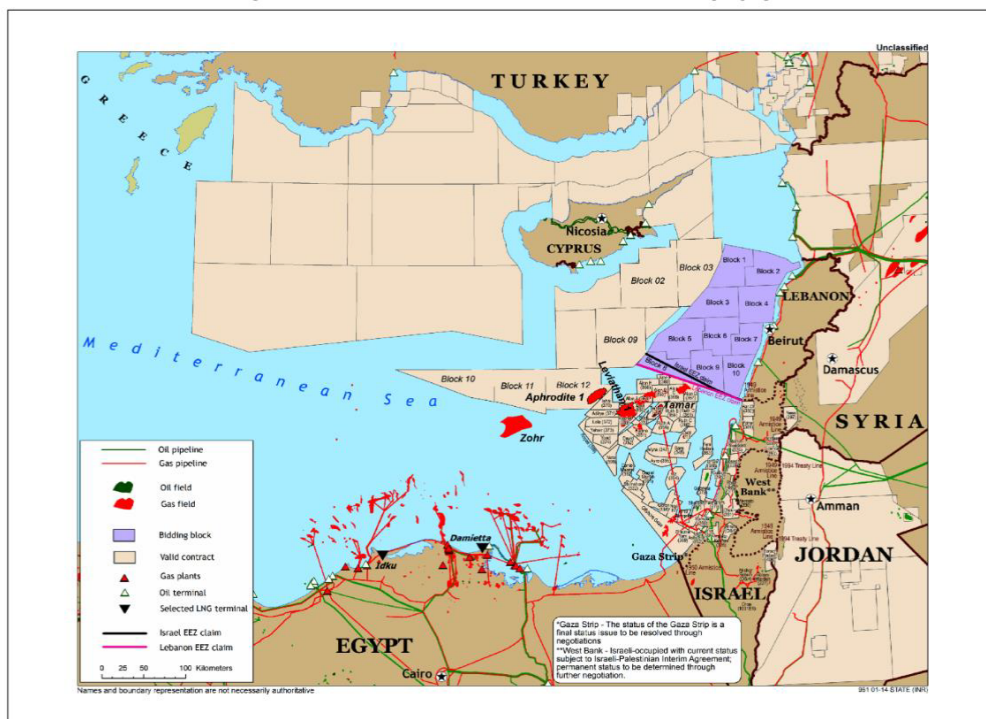
Εικόνα 3: Γεωγραφία υποδομών και δικτύων πετρελαίου και Φ/Α Αν.Μεσογείου
