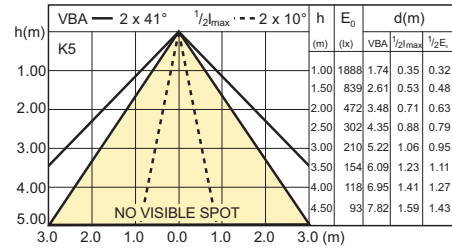
5.5-50W E27 3000K PAR20 25D
