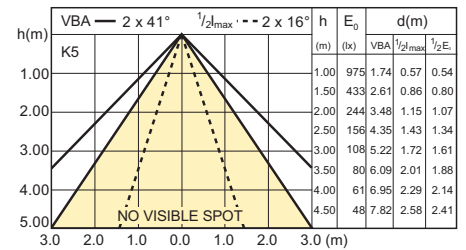
5.5-50W E27 4000K PAR20 40D
