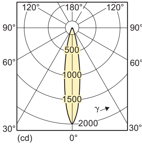
5.5-50W E27 4000K PAR20 25D
