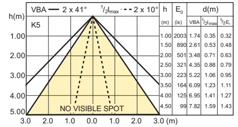
5.5-50W E27 4000K PAR20 25D
