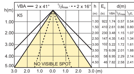
5.5-50W E27 3000K PAR20 40D
