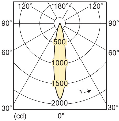
5.5-50W E27 3000K PAR20 25D
