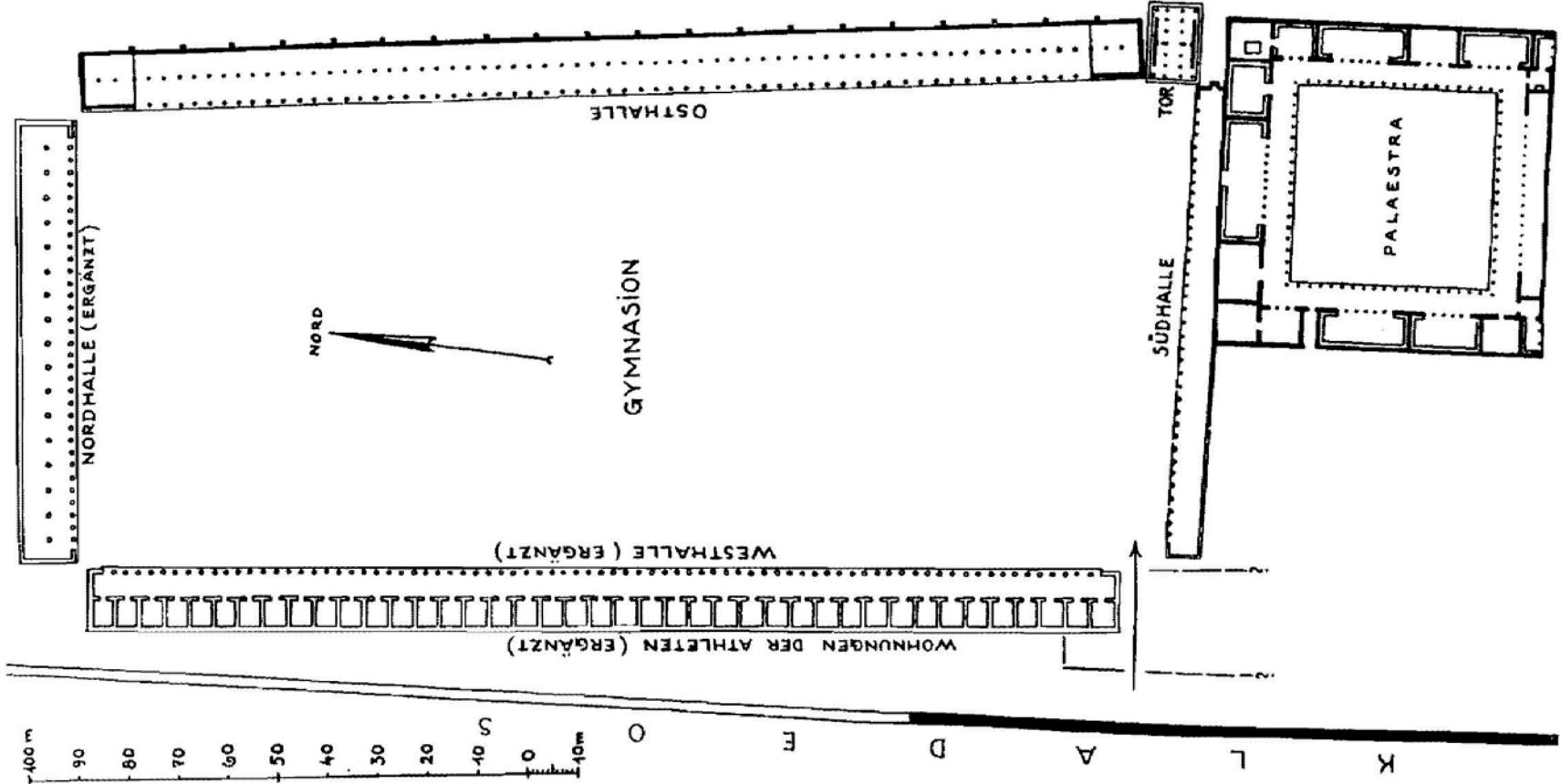
Abb. 3 Rekonstruierter Grundriß der Platzanlage des Gymnasium
