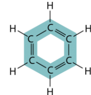
Βενζόλιο
