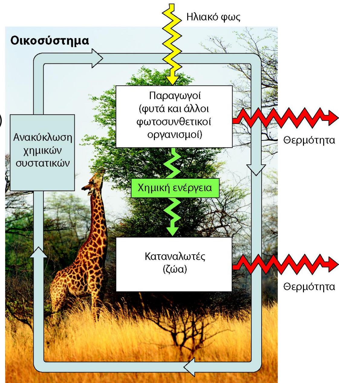
▲ Εικόνα 1.5 Ανακύκλωση θρεπτικών υλών και ροή ενέργειας σε ένα οικοσύστημα.
