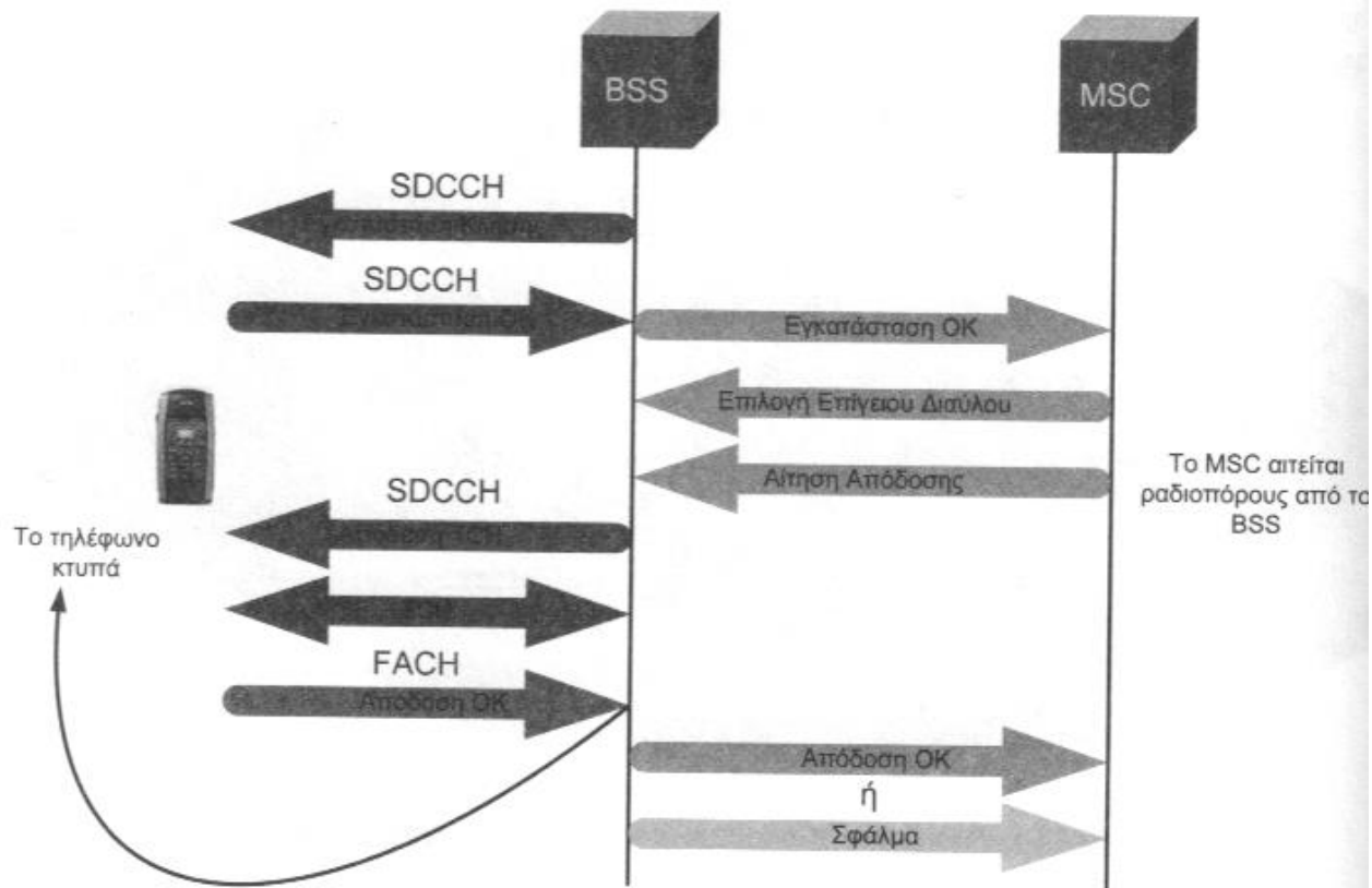
Σχήμα 6.47: Διαδικασία εγκατάστασης κλήσης
