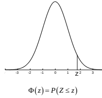
Πίνακας 6. Τυποποιημένη Κανονική Κατανομή (συνέχεια)
