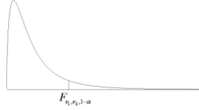
Πίνακας 9. Ποσοστιαία Σημεία της Κατανομής F (συνέχεια)
