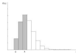
Πίνακας 5. Αθροιστικές Πιθανότητες Κατανομής Poisson
